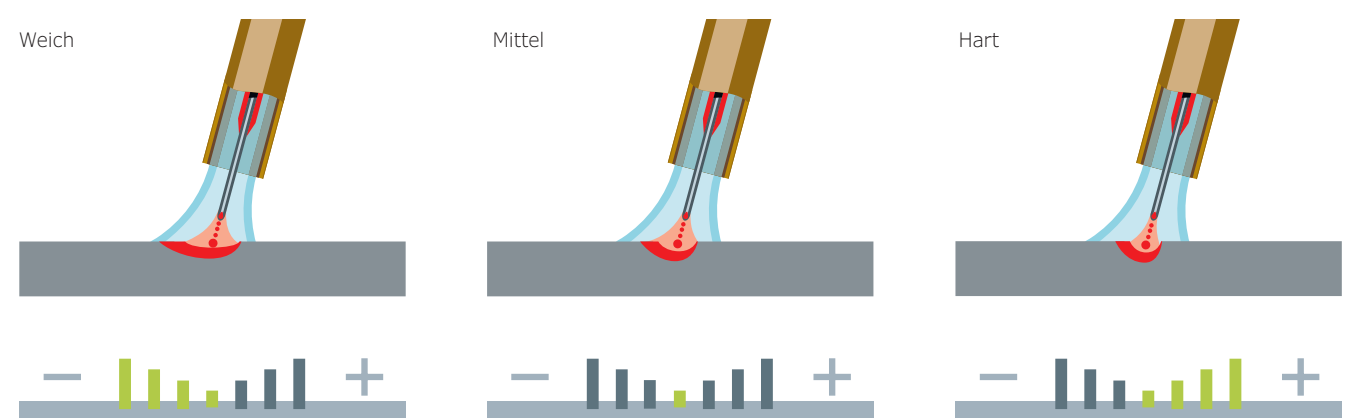
Die Dynamikregelung ermöglicht einen breiteren oder schmalen Lichtbogen – wie es dem Schweißer beliebt.
