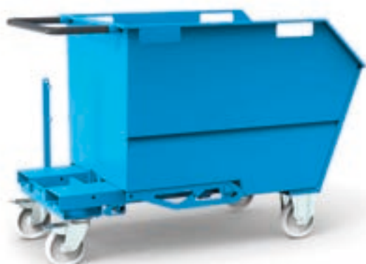
Benna portarottami ribaltabile capacità 500 L con ruote predisposta per griglia e rubinetto
