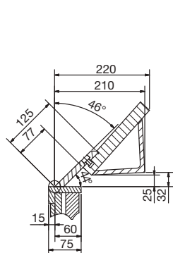
Dimensioni E-Serie
